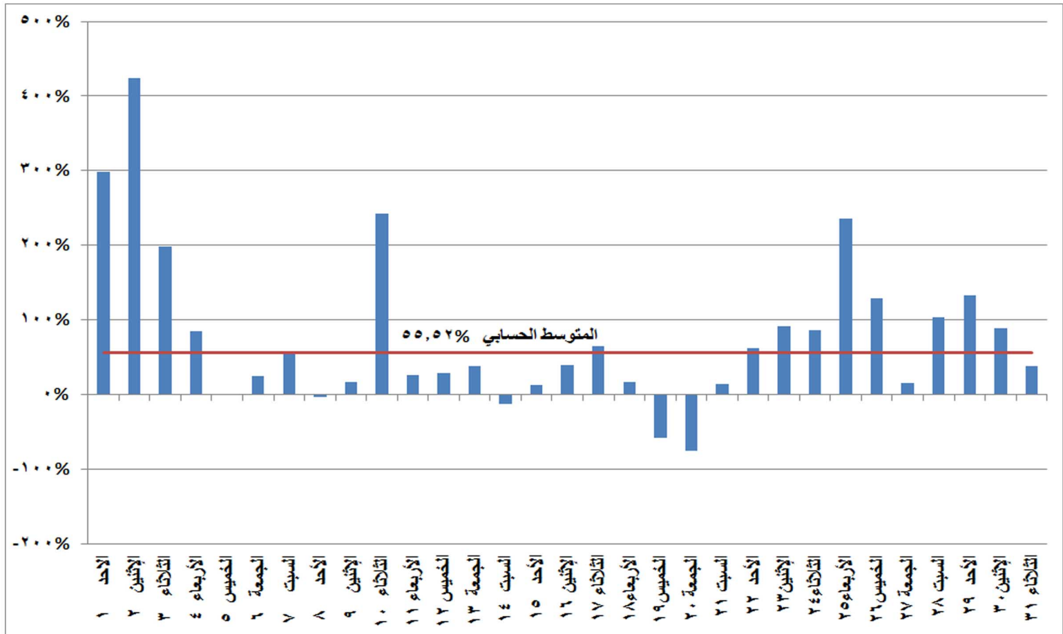
شكل (٢٦) نسب التغير في استخدام الرياح والشمس في إنتاج الطاقة الكهربائية خلال شهر مارس ٢٠٢٠ مقارنة بالشهر المماثل من العام السابق
