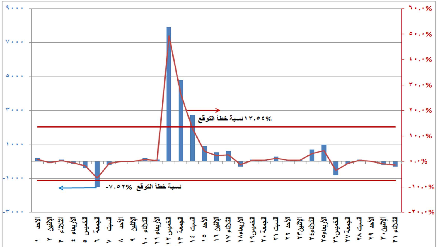
شكل (١٠) الفرق بين الحمل الأقصى المتوقع والمسجل فعليا ونسبة الفرق إلى الحمل المسجل فعليا خلال شهر مارس ٢٠٢٠
