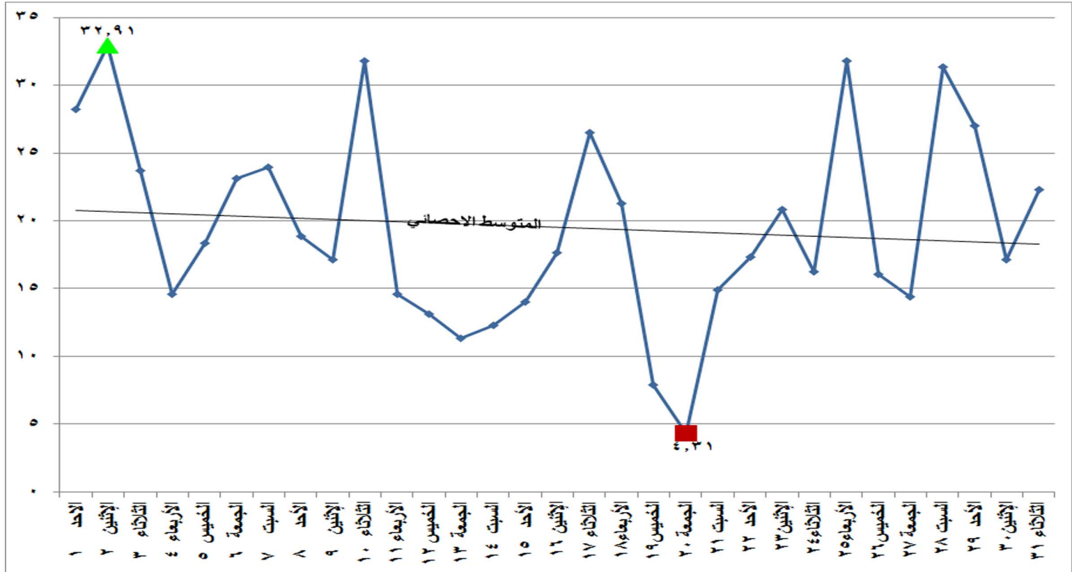
شكل (٢٥) الطاقة الكهربائية المنتجة من الرياح والشمس خلال شهر مارس ٢٠٢٠
