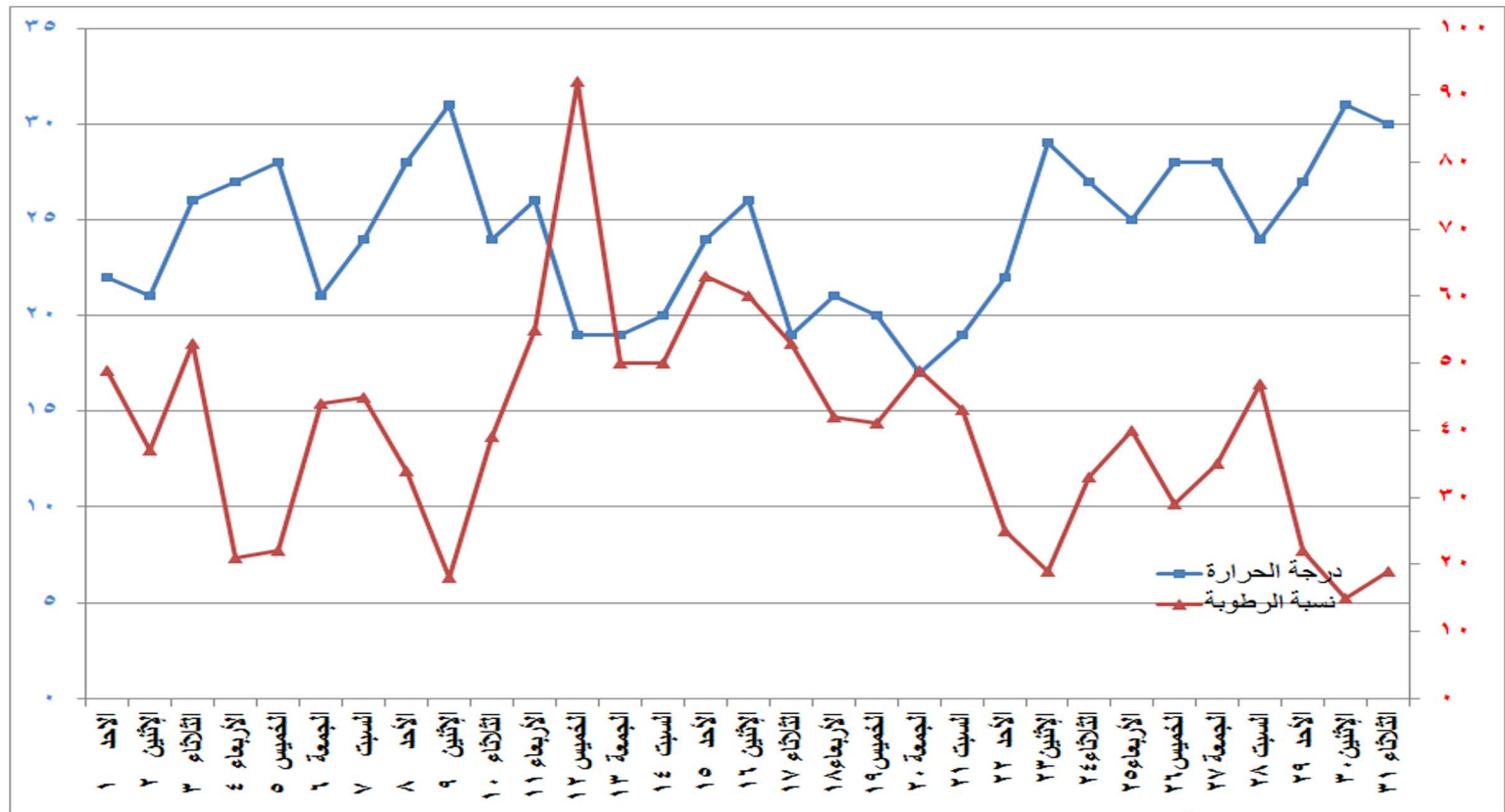
شكل (١١) التغيير في درجة الحرارة والرطوبة النسبية خلال شهر مارس ٢٠٢٠
