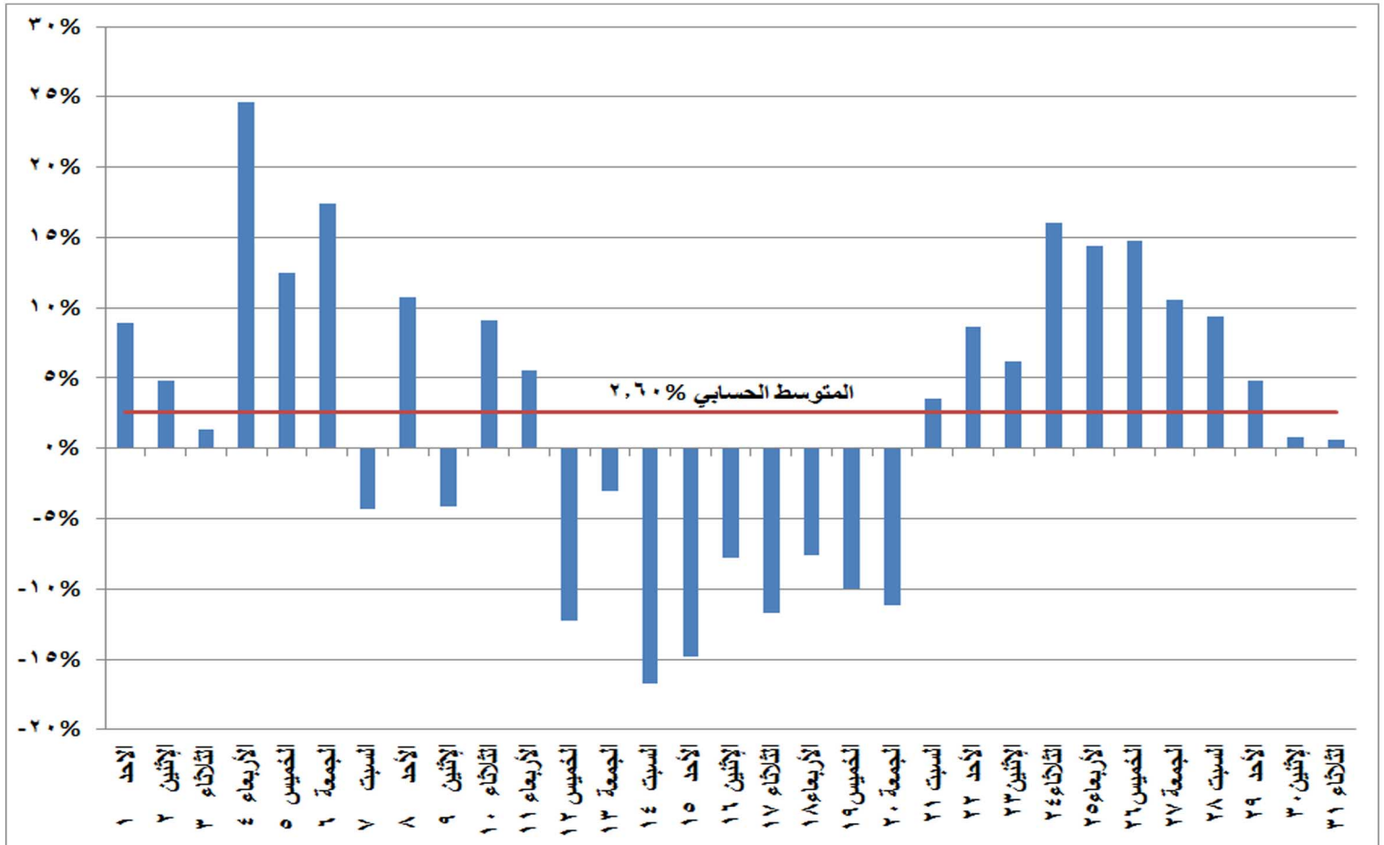
شكل (٢٤) نسب التغير في استخدام المصادر المائية في إنتاج الطاقة الكهربائية خلال شهر مارس ٢٠٢٠ مقارنة بالشهر المماثل من العام السابق
