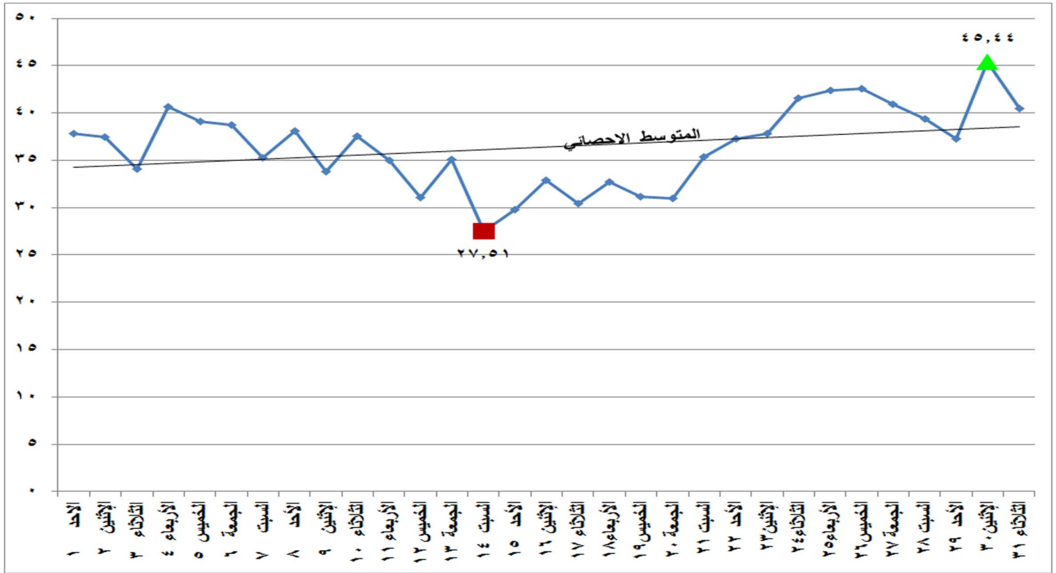
شكل (٢٣) الطاقة الكهربائية المنتجة من المصادر المائية خلال شهر مارس ٢٠٢٠
