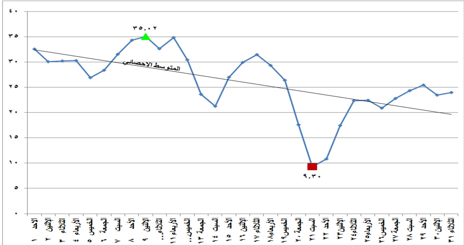
شكل (١٩) الطاقة الكهربائية المنتجة من المازوت خلال شهر مارس ٢٠٢٠
