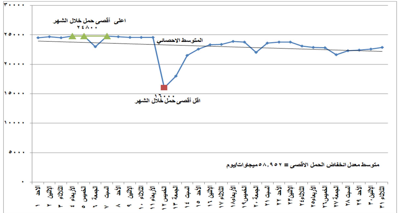
شكل (١) تطور الحمل الاقصى اليومي خلال شهر مارس ٢٠٢٠
