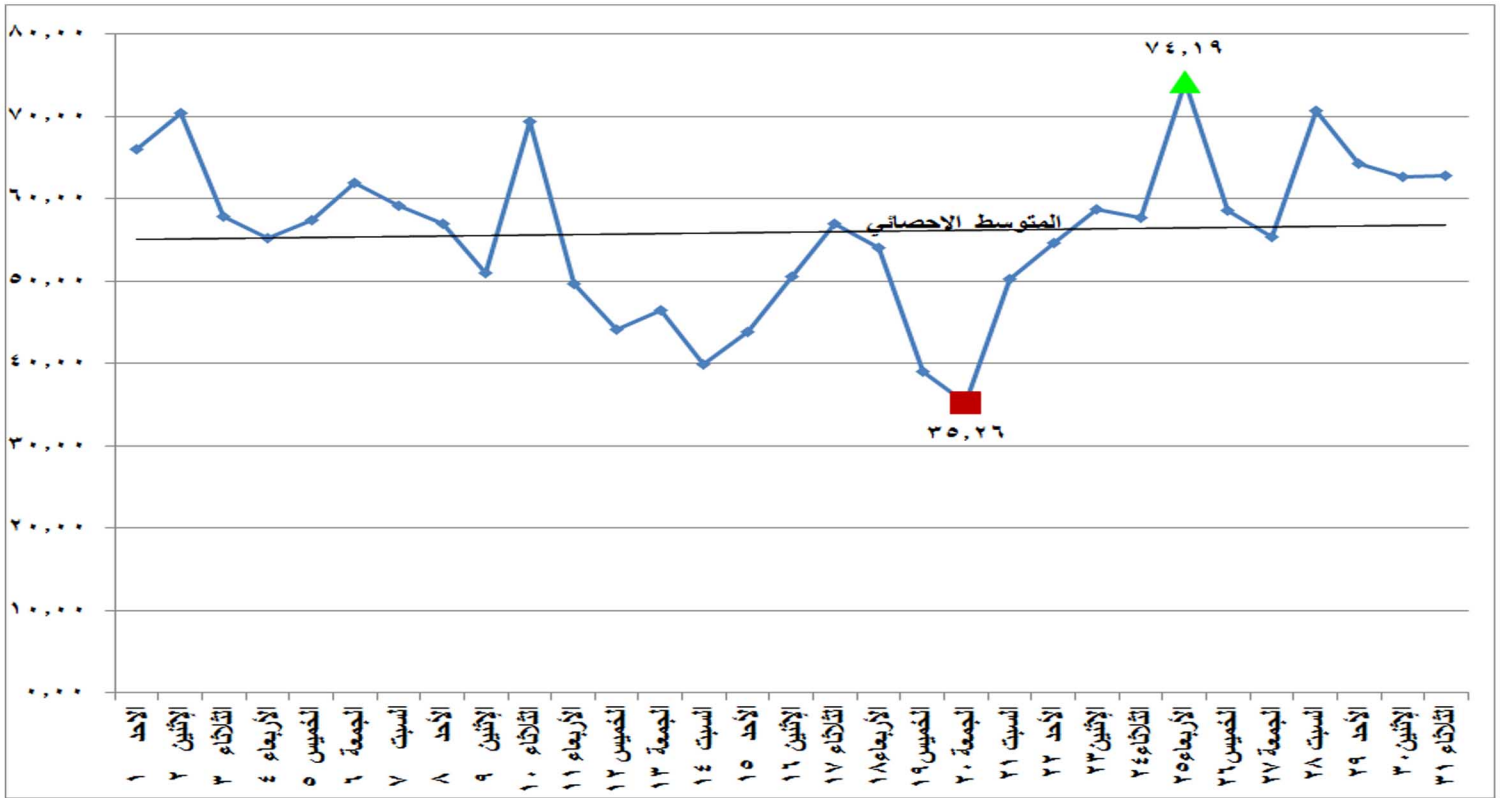
شكل (٢١) الطاقة الكهربائية المنتجة من المصادر غير الحرارية خلال شهر مارس ٢٠٢٠
