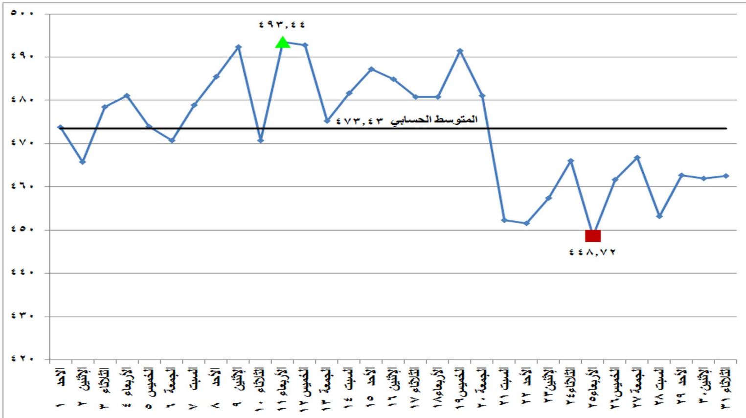
شكل (١٤) معامل انبعاثات غاز ثاني اكسيد الكربون المكافئ على مدى شهر مارس ٢٠٢٠
