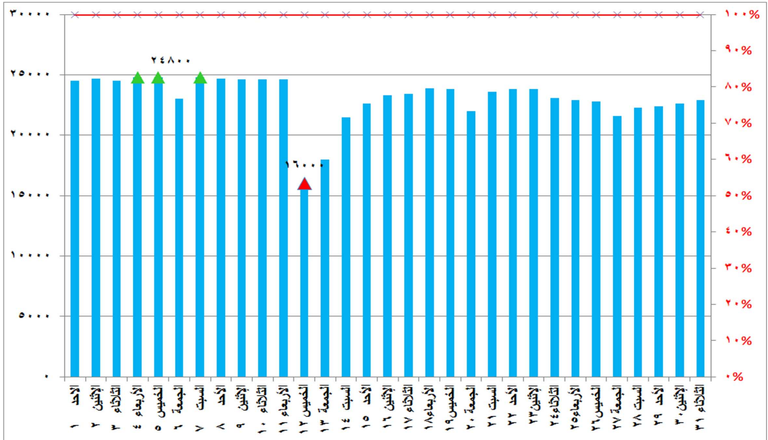
شكل (٥) قدرات الانتاج المتاحة ونسبتها للحمل الاقصى خلال شهر مارس ٢٠٢٠
