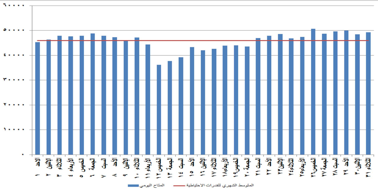
شكل (٢٧) القدرات المتاحة يوميا والمتوسط الشهري للقدرة الاحتياطية خلال شهر مارس ٢٠٢٠
