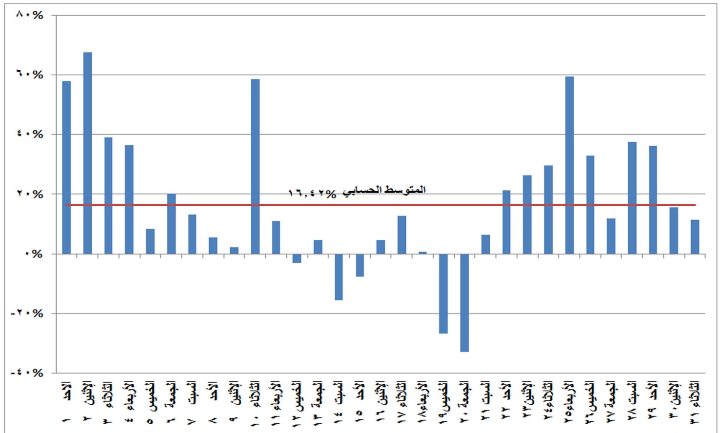
شكل (٢٢) نسب التغير في استخدام المصادر غير الحرارية في إنتاج الطاقة الكهربائية خلال شهر مارس ٢٠٢٠ مقارنة بالشهر المماثل من العام السابق
