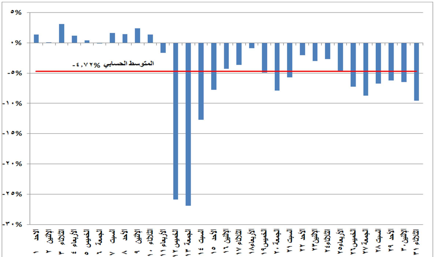
شكل (١٦) نسب التغير في الطاقة الكهربائية المنتجة خلال شهر مارس ٢٠٢٠ مقارنة بالشهر المماثل من العام السابق
