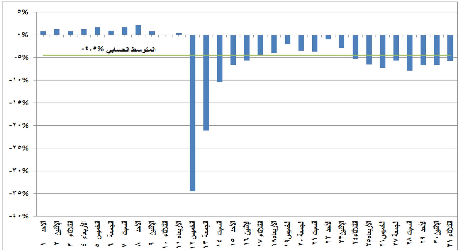
شكل (٩) النسب المئوية للتغير في الحمل الاقصى خلال شهر مارس ٢٠٢٠ مقارنة باليوم المماثل من العام الماضي
