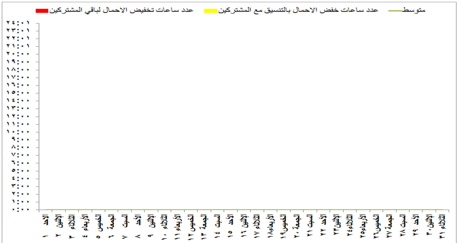
شكل (٤) عدد الساعات التي تجاوزت فيها الاحمال قدرات الانتاج المتاحة خلال شهر مارس ٢٠٢٠
