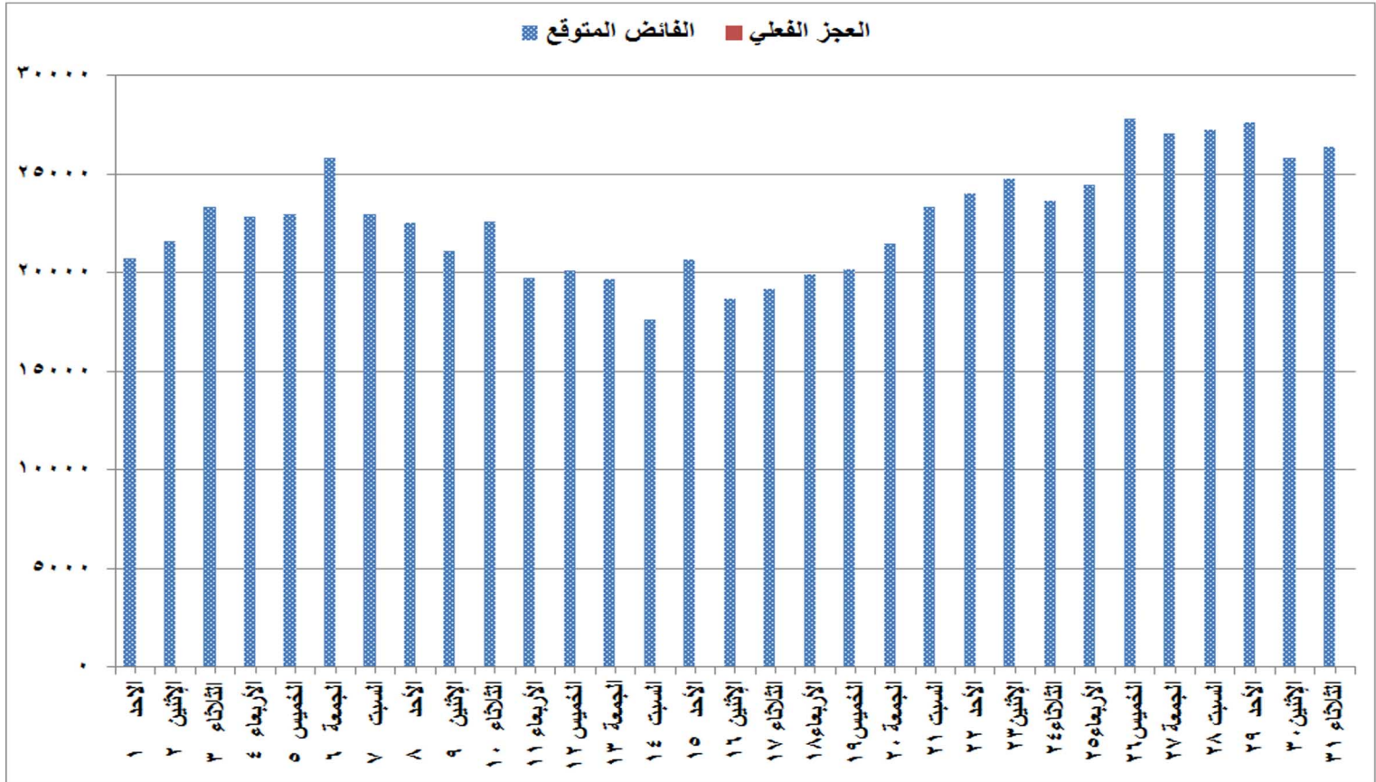
شكل (٧) الفائض والعجز المتوقع للقدرات خلال شهر مارس ٢٠٢٠
