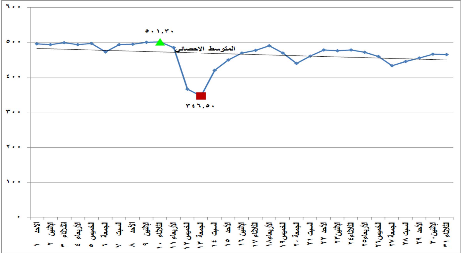
شكل (١٥) إجمالي الطاقة الكهربائية المنتجة من كل المصادر الأولية خلال شهر مارس ٢٠٢٠
