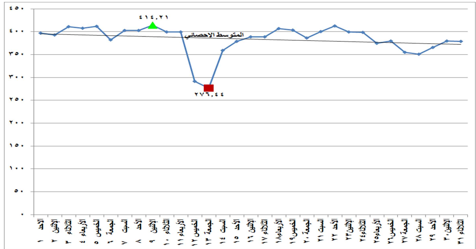
شكل (١٧) الطاقة الكهربائية المنتجة من الغاز الطبيعي خلال شهر مارس ٢٠٢٠
