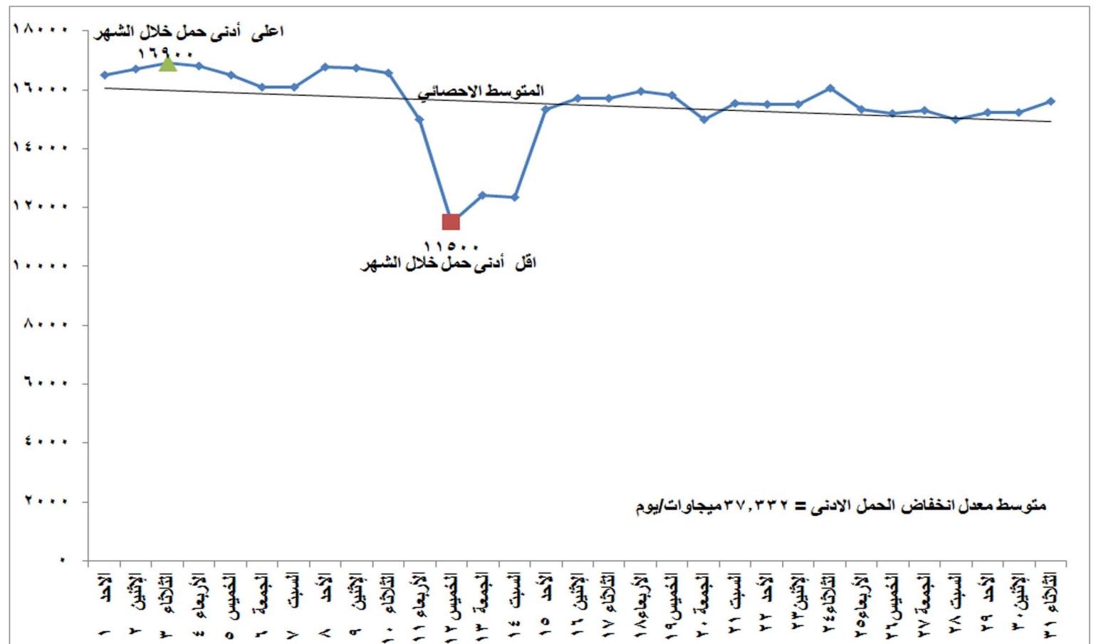
شكل (٢) تطور الحمل الادنى اليومي خلال شهر مارس ٢٠٢٠
